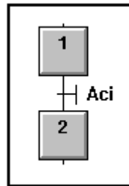
Ilustración 2- Representación literal de la receptividad
