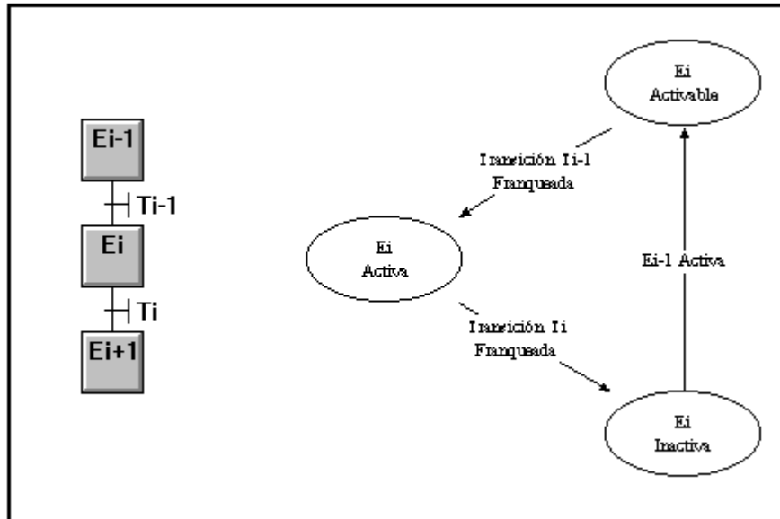
Ilustración 4- Estados posibles de la etap Ei y sus transiciones
