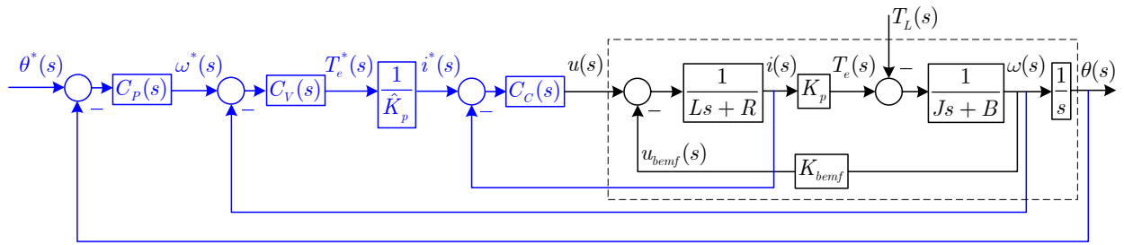
Figura 2: Control en cascada del motor de corriente continua.
